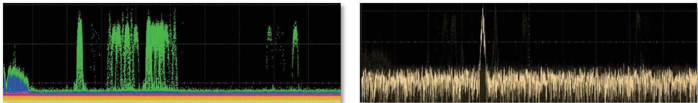
突发的蓝牙数据很难通过标准 FFT 持续捕获（右图），但在 RTSA 下则无所遁形（左图）。
